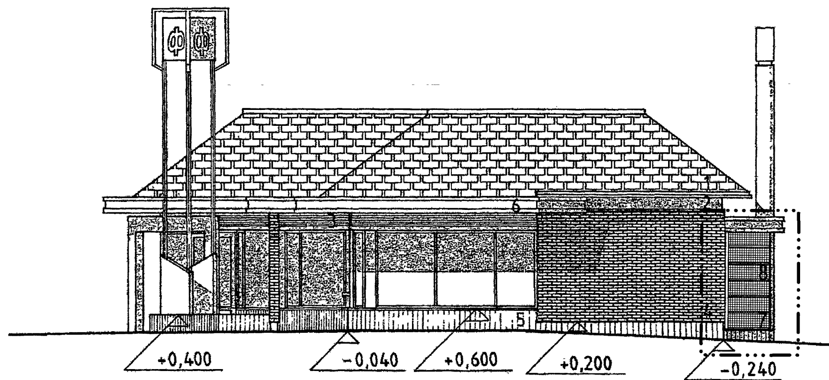
JULKISIVU KOIVISTONTIELLE
