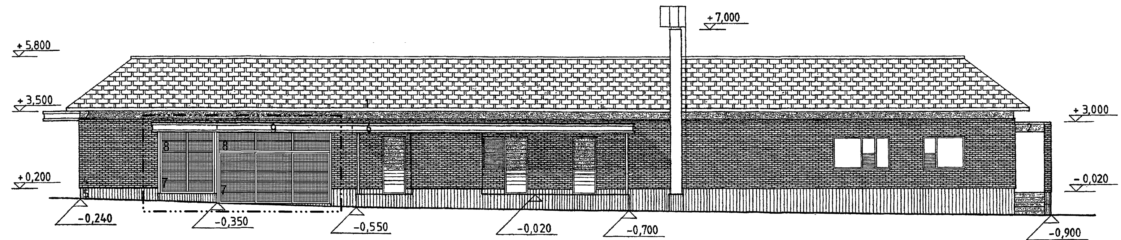
JULKISIVU TAKAPIHALLE
