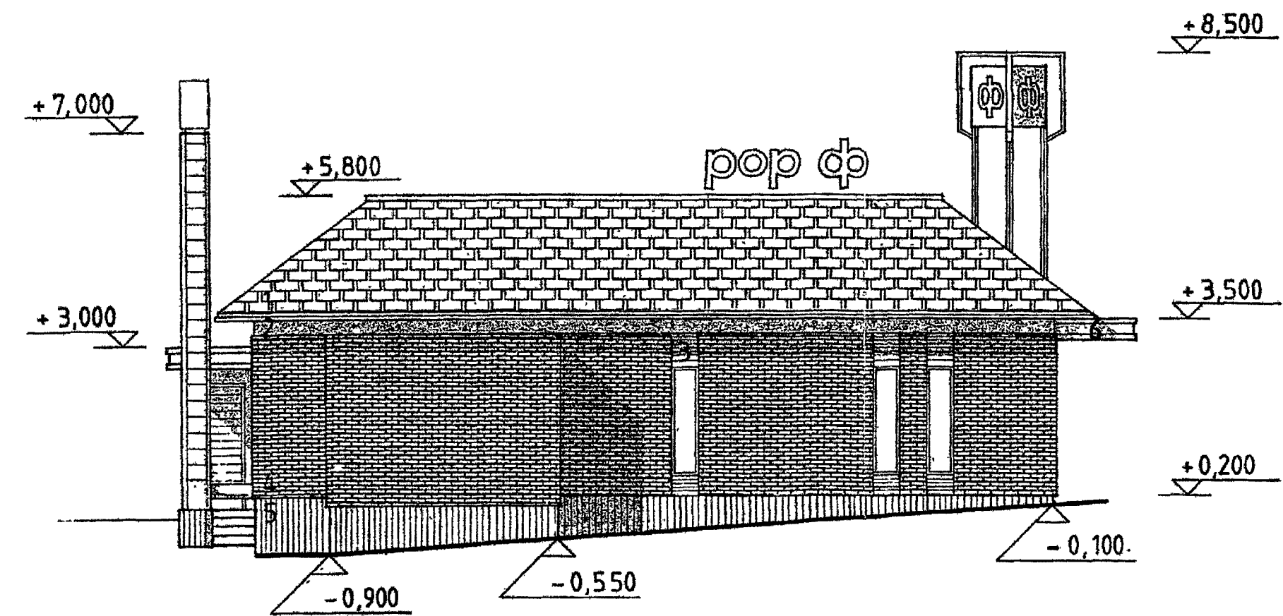
JULKISIVU TAMPEREENTIELLE
